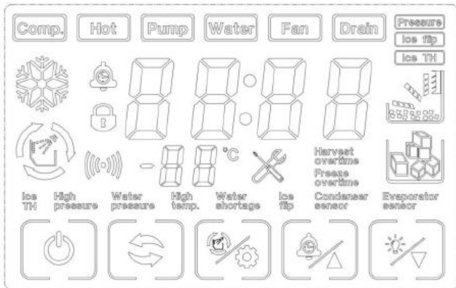
Рис4 Панель управления (сенсорная)
